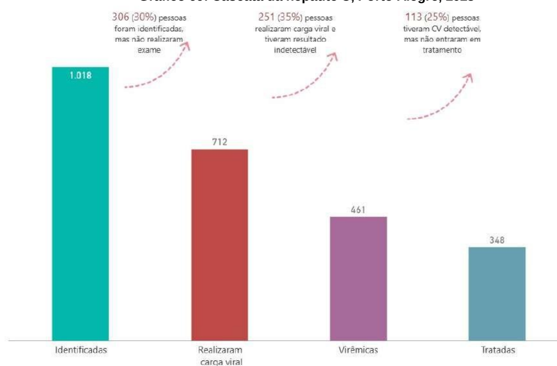
Gráfico 69: Cascata da hepatite C, Porto Alegre, 2023
