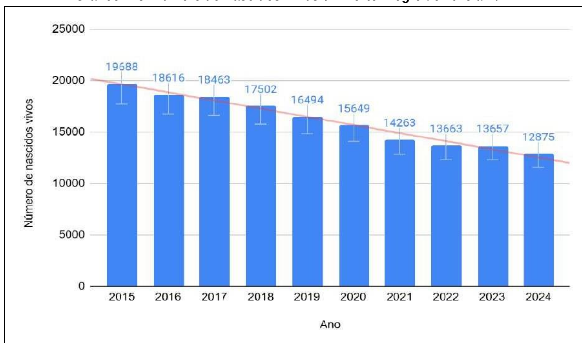
Gráfico 178: Número de Nascidos Vivos em Porto Alegre de 2015 a 2024
