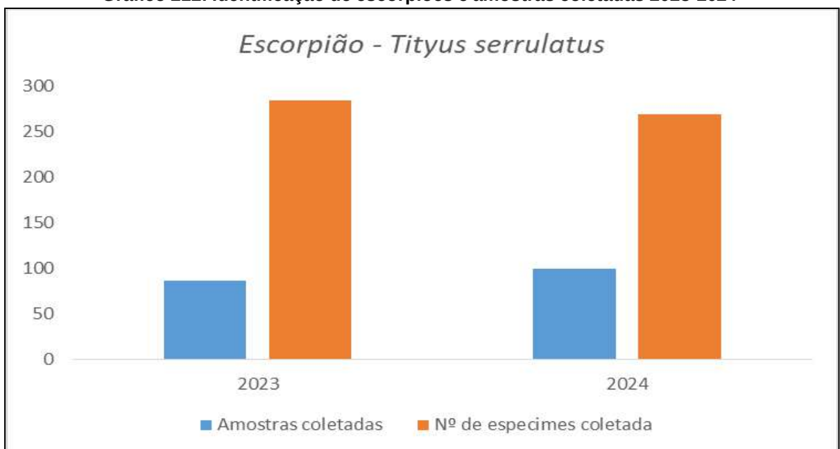
Gráfico 212: Identificação de escorpiões e amostras coletadas 2023-2024
