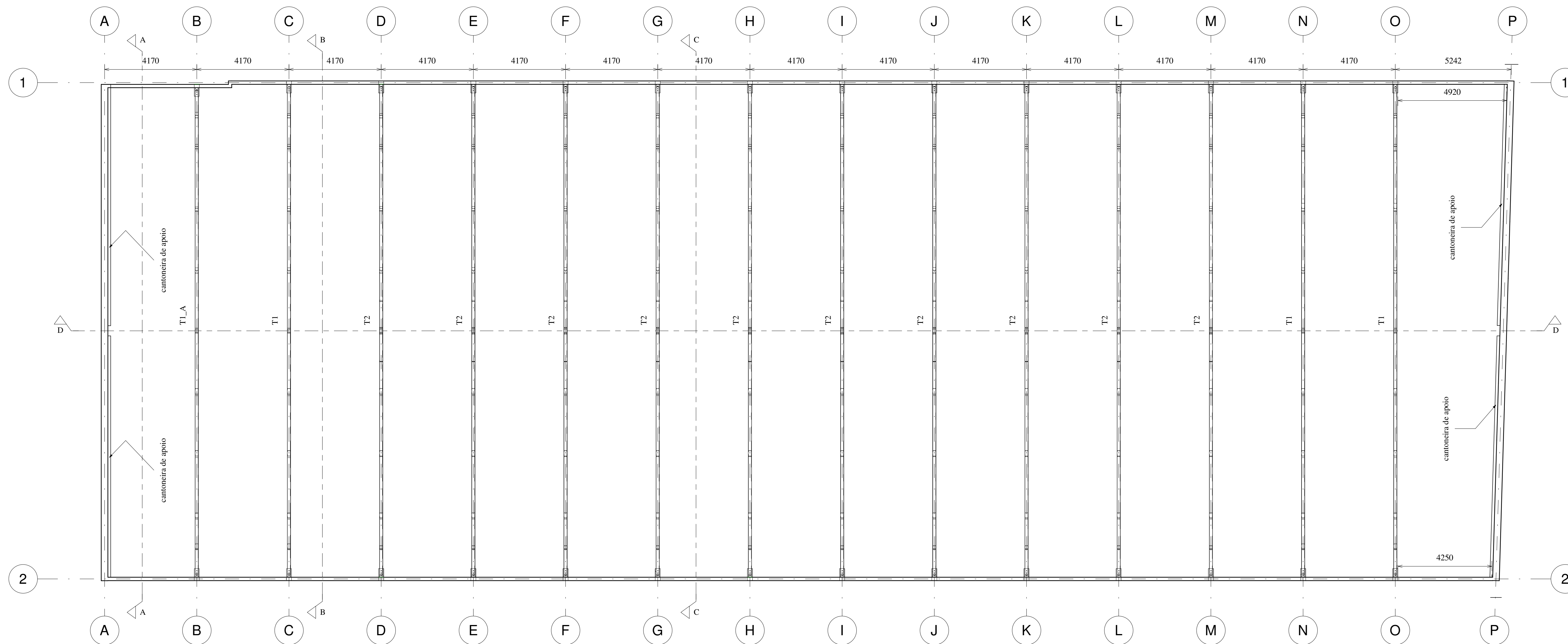
Locação Tesouras e Cantoneiras de apoio 1 : 100
