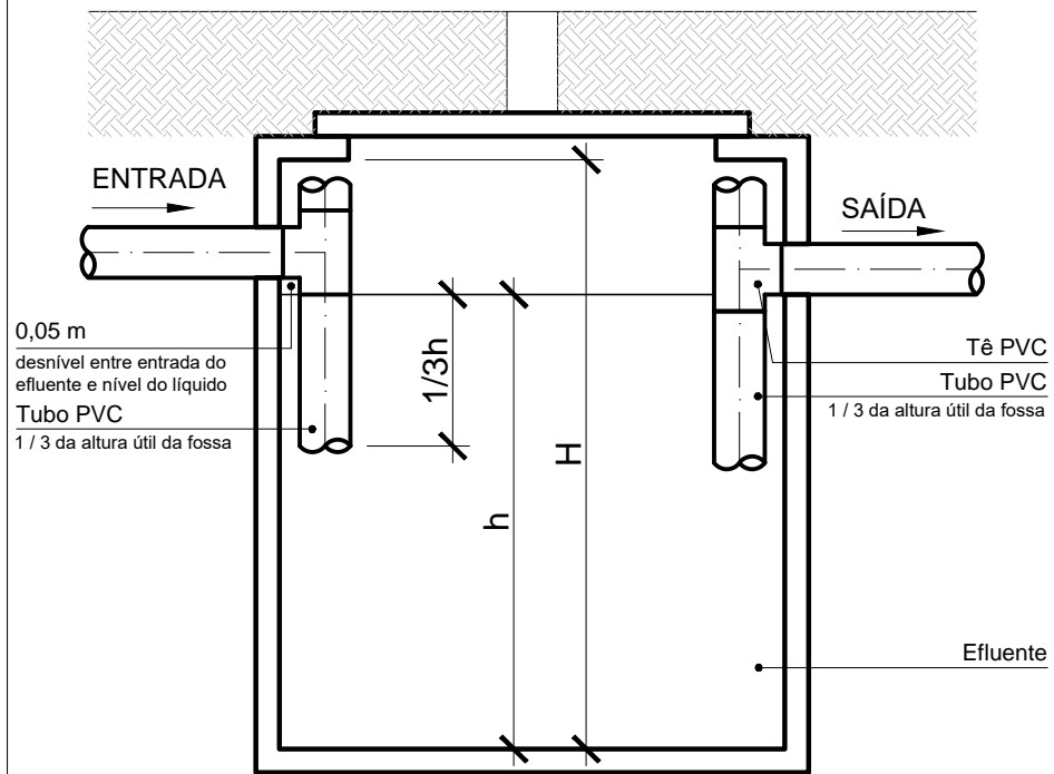
FOSSA SEPTICA
