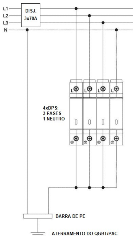
Figura 1: Ligação de DPS na instalação do QGBT/PAC da EBE Irmãos Maristas II. A ligação supra também serve de referência para o QAP-GM.
