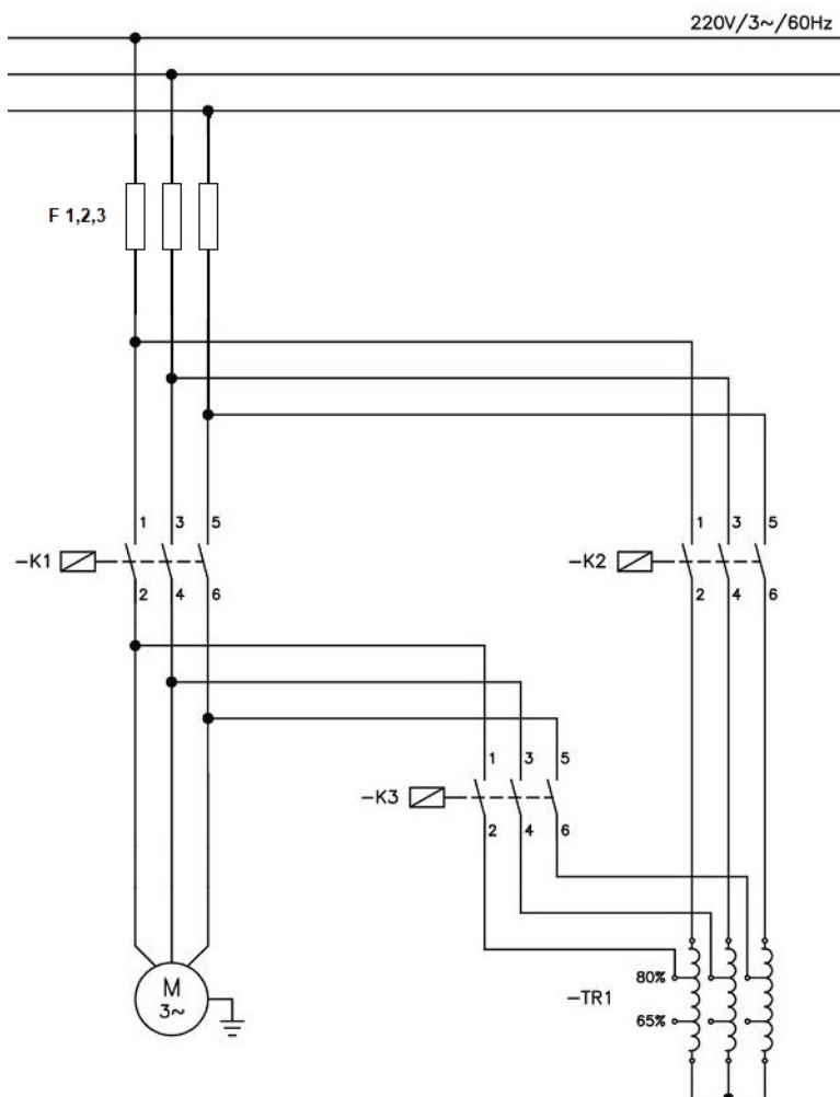
Figura 2: diagrama referencial trifilar de montagem para chave de partida autocompensadora.
