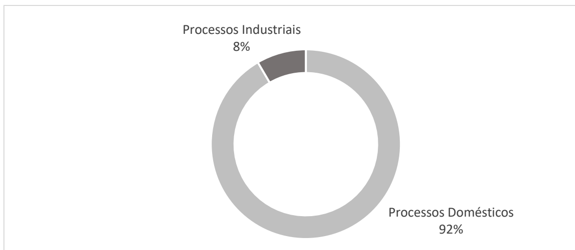
Figura 14. Análise da componente cinza da pegada hídrica por processo.
