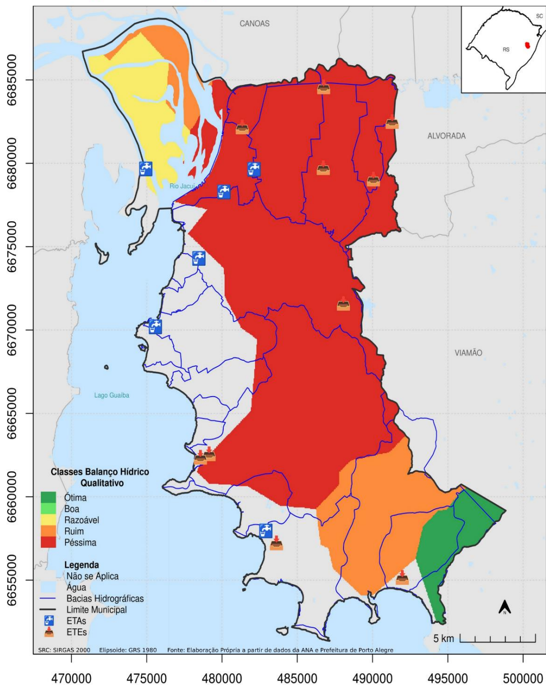
Figura 25. Balanço Hídrico Qualitativo do município de Porto Alegre.
