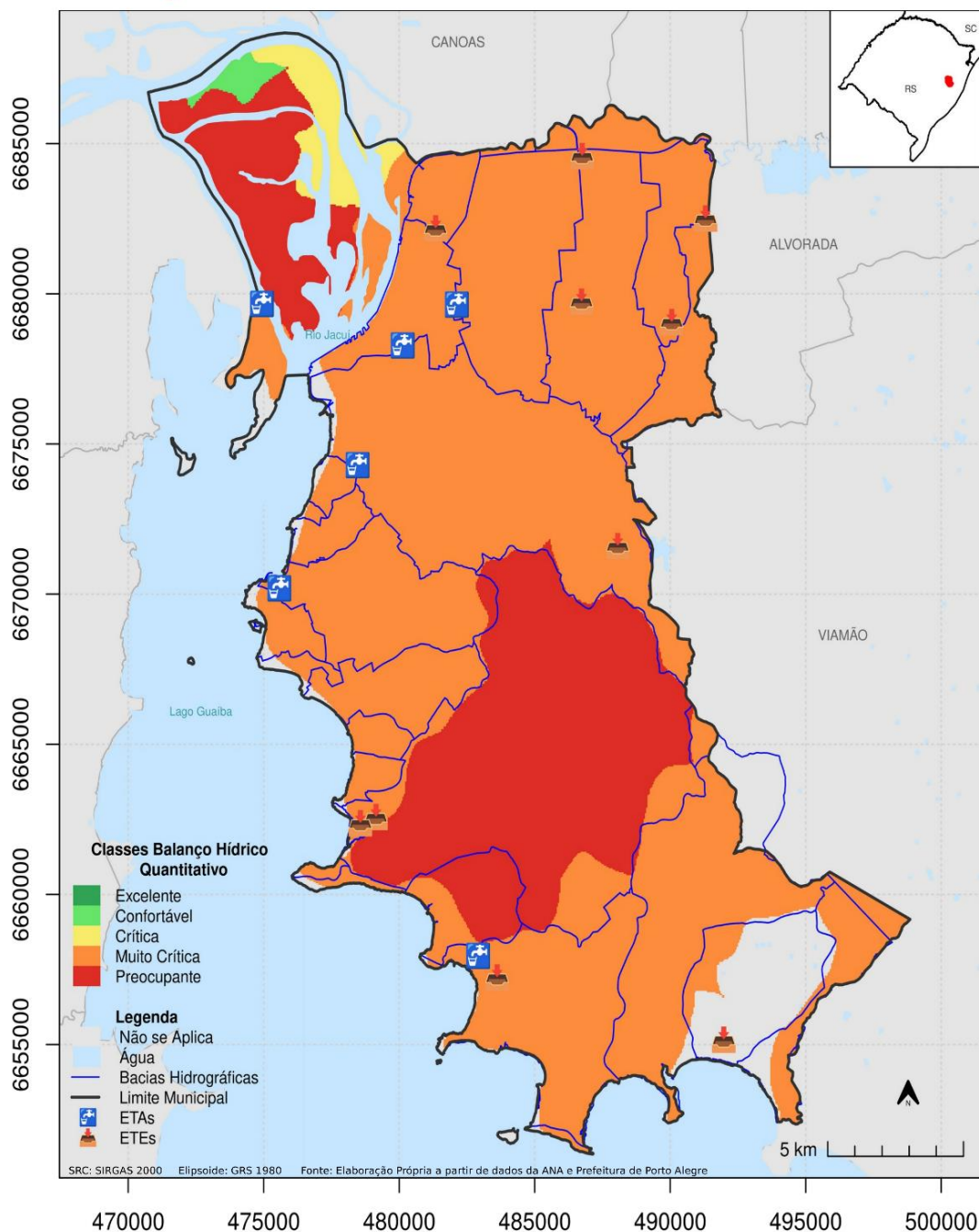
Figura 24. Balanço Hídrico Quantitativo do município de Porto Alegre.
