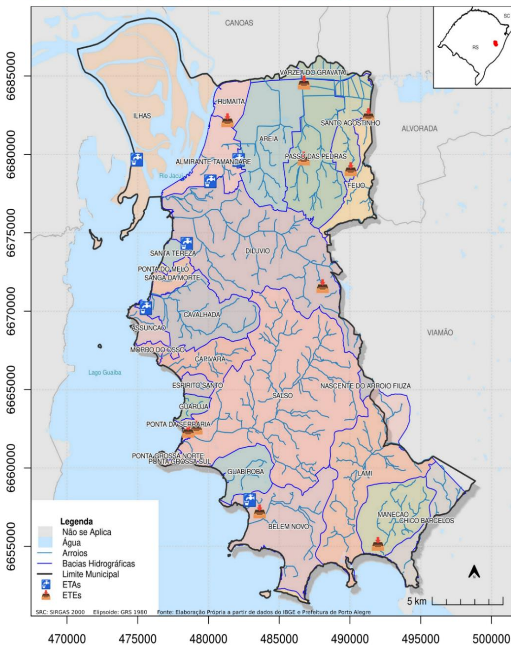
Figura 3. Mapa de sub-bacias hidrográficas, arroios, e localização de estações de tratamento de água e efluentes de Porto Alegre.
