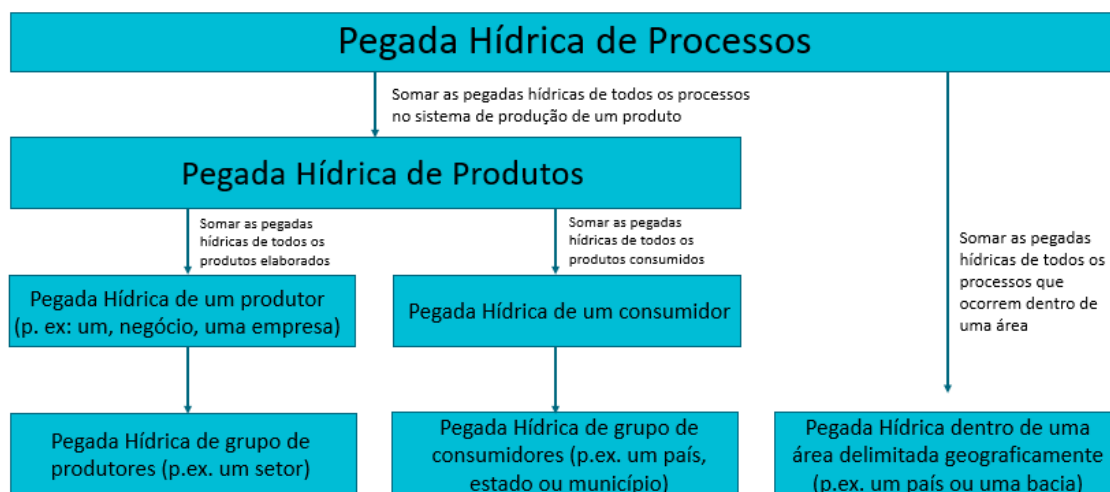
Figura 10. Pegada hídrica de processos como a unidade básica para todas as outras pegadas hídricas.
