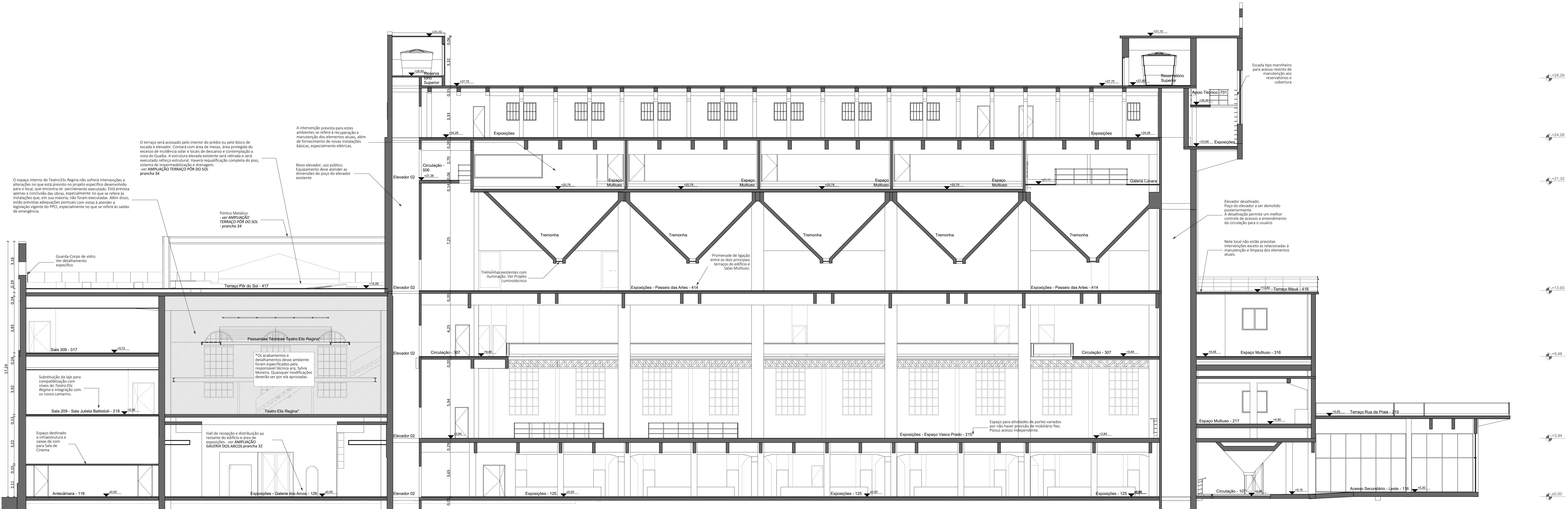
CORTE AA 1:100
