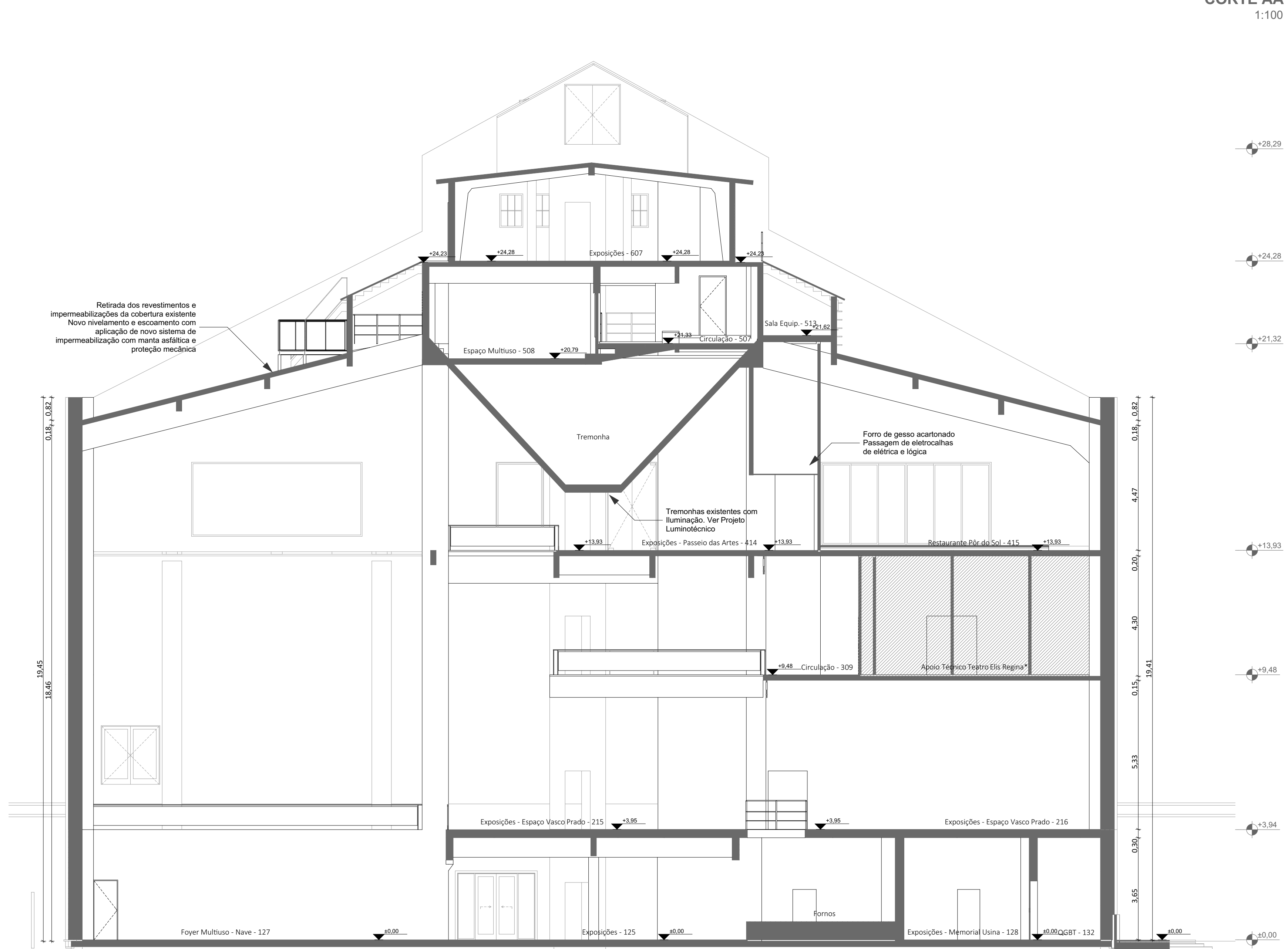
CORTE CC 1:100
