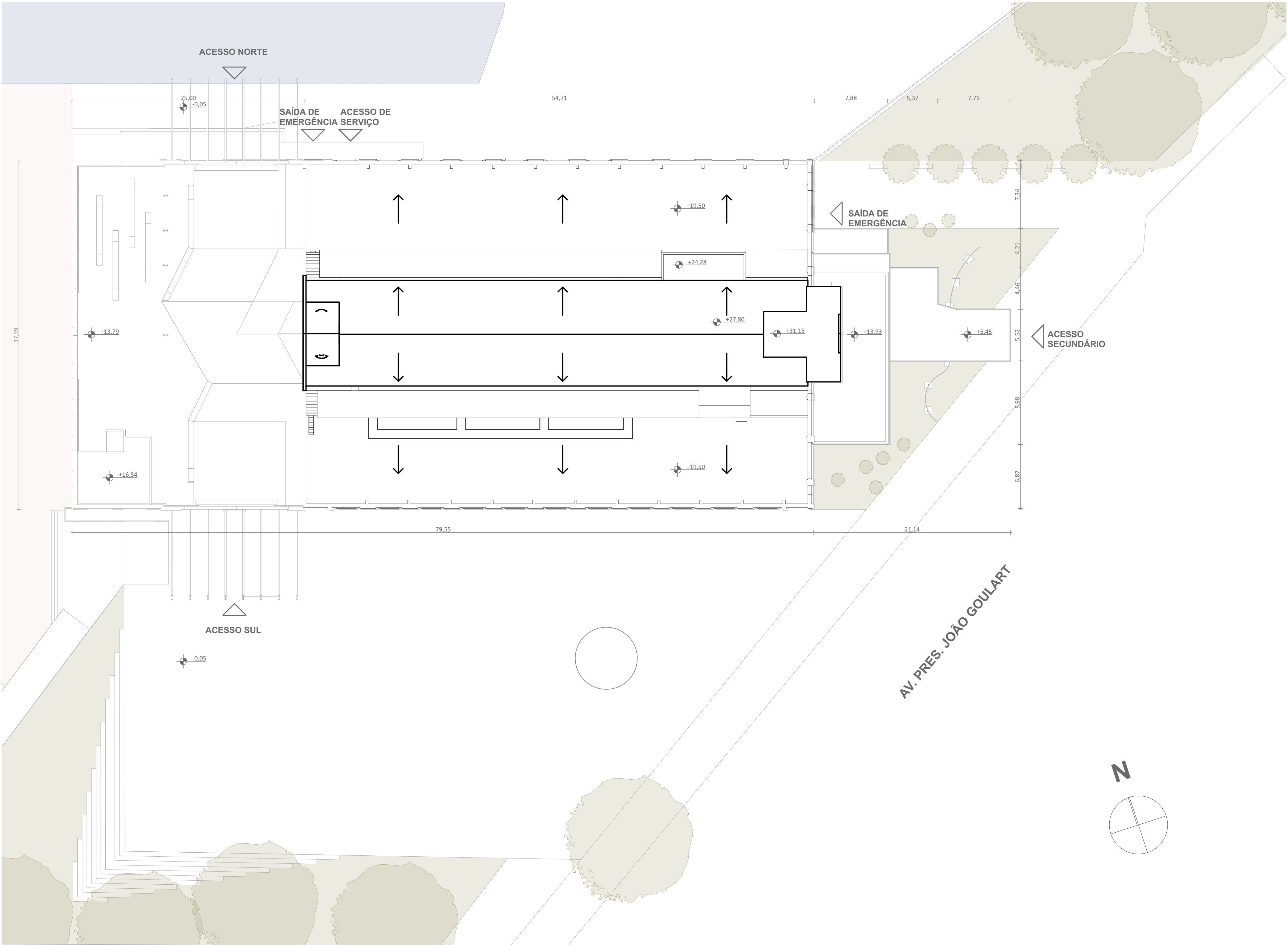
IMPLANTAÇÃO 1:250
