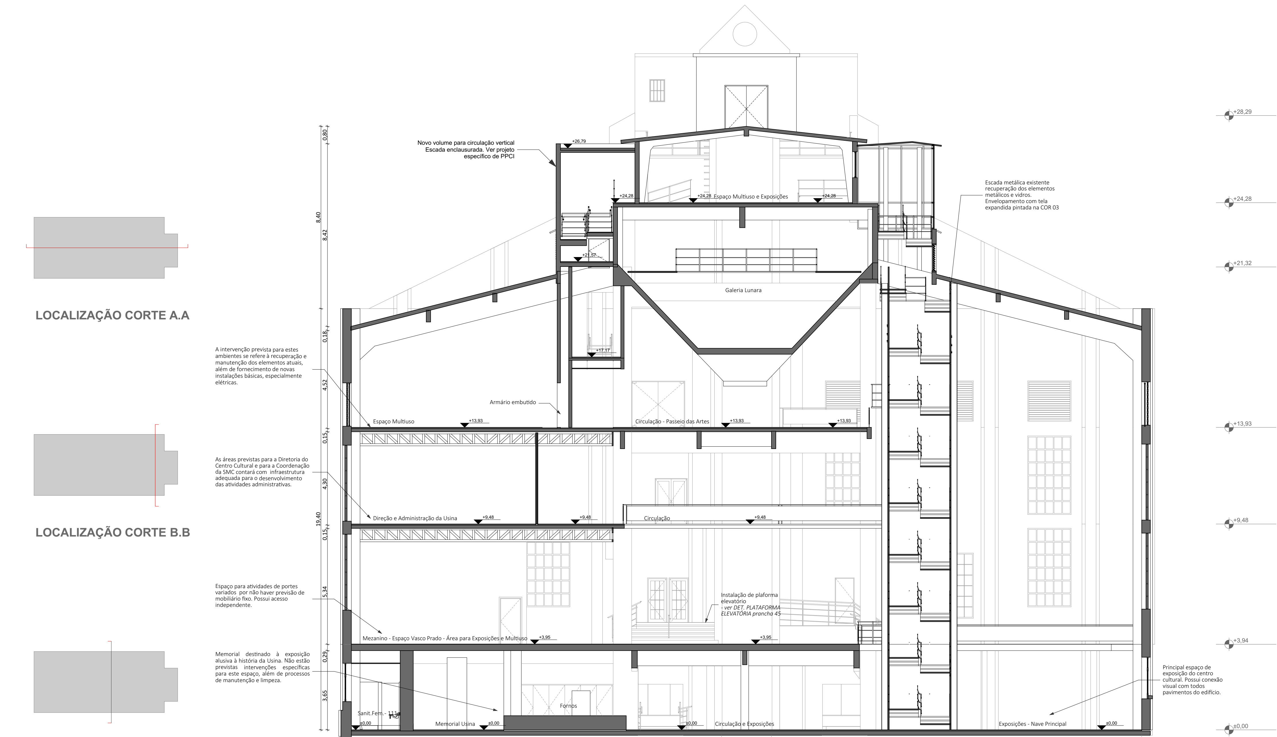
CORTE BB 1:100
